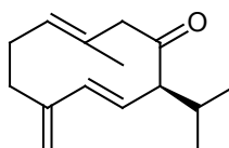
germacrone
