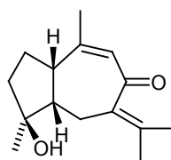
epiprocurcumenol
