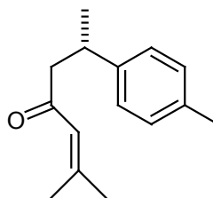
ar -turmerone
