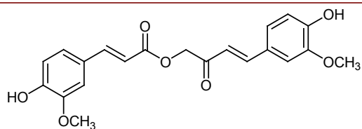
calebin-A
