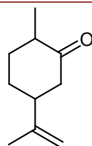
piperitone
