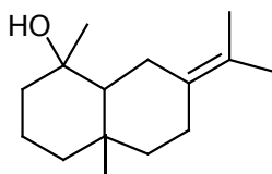
juniper camphor
