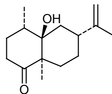
corymbolone
