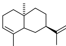
\alpha -selinene
