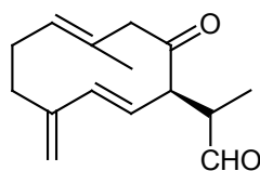
germacrone-13-al
