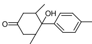
curcuma-J
