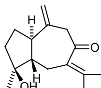
isoprocurcumenol
