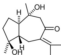
zedoaronediol
